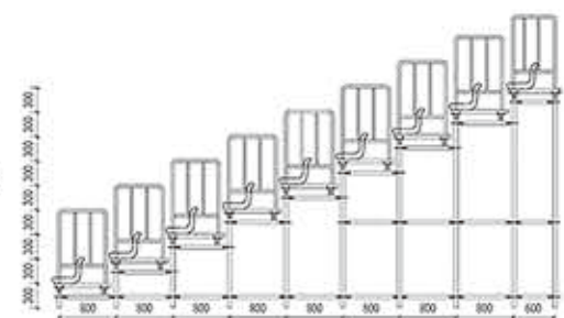
SJ-A032 拆装式看台 SJ-A032 Detachable Telescopic Grandstand
